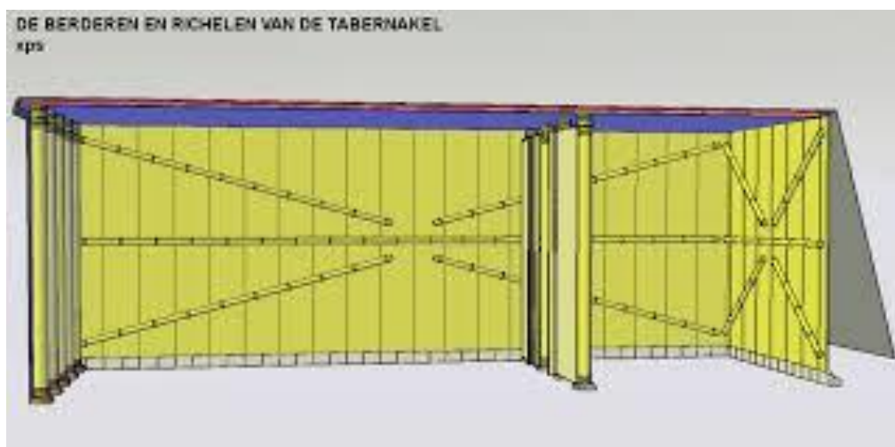
De berderen en richels (= dwarsbalken) van de tabernakel
